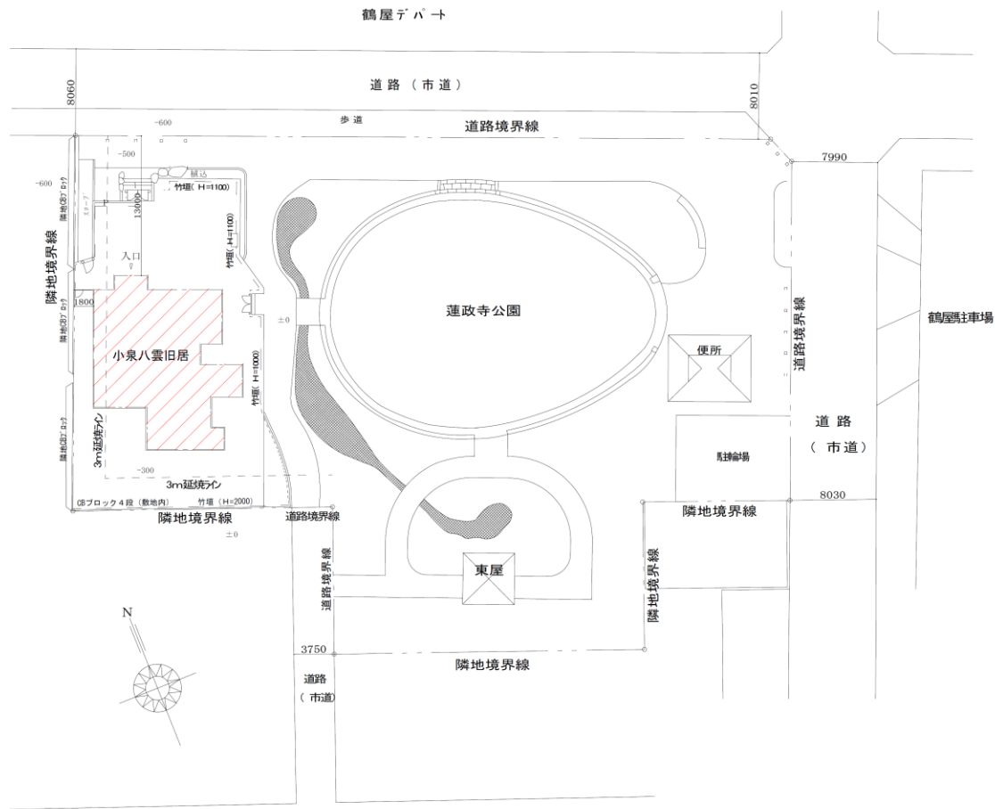
全体配置図 S=1/400
