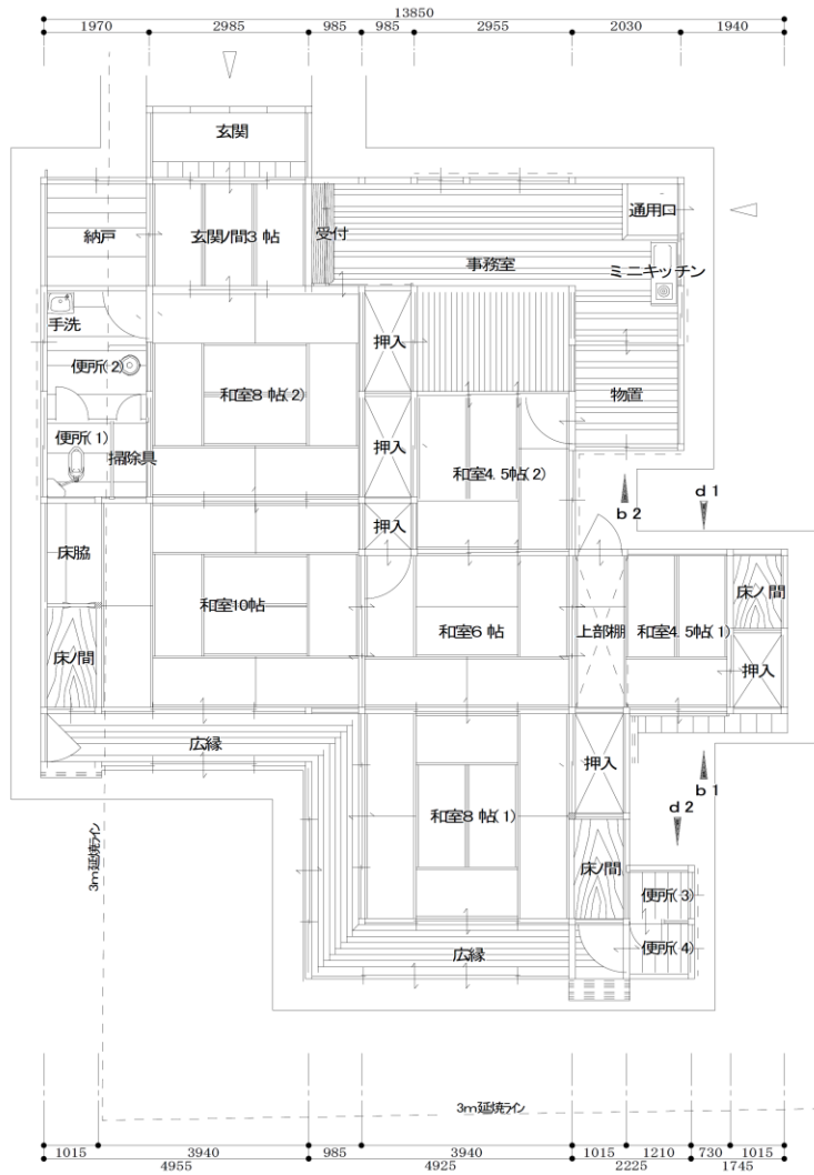
平面図 S=1/100
