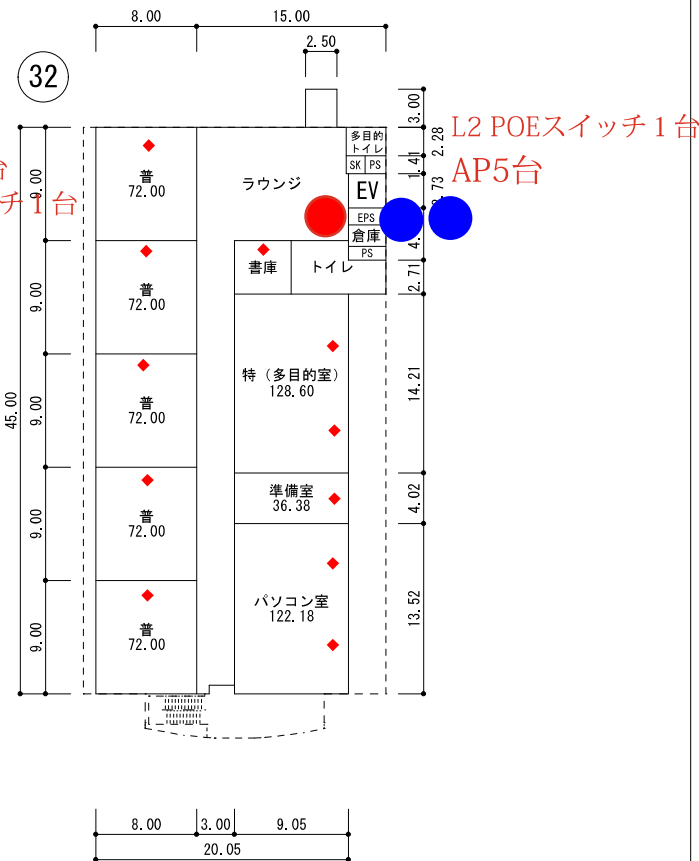
【第32棟：3階平面図】
