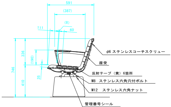
断面図
