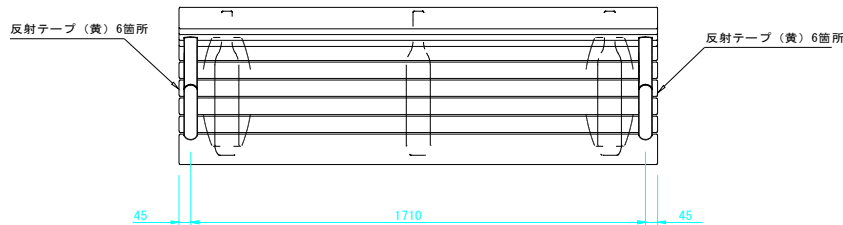
正面図
