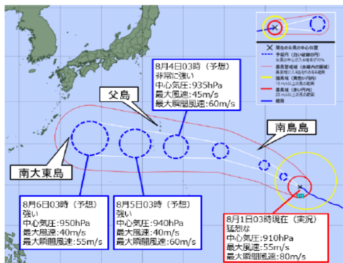
■ 台風情報(台風第13号)[8月1日03時]
