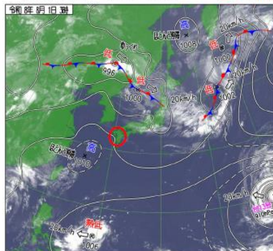
地上天気図（1日3時）
