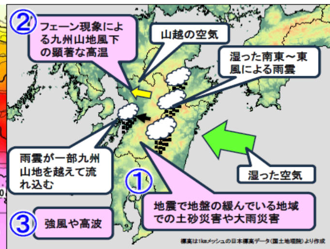
■ 台風が沖縄・奄美に進んだ場合の起こりうる現象のイメージ
