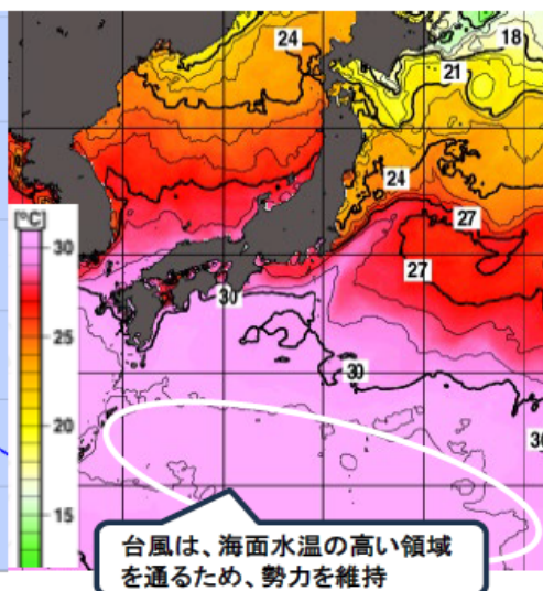
■ 海面水温[7月30日]
