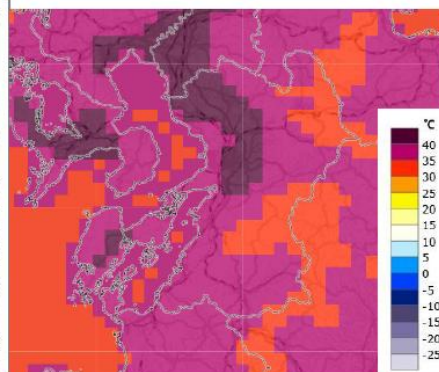
3日日中の最高気温（予想）
