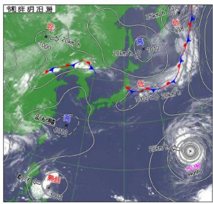
衛星赤外画像と地上天気図 (2日3時)
