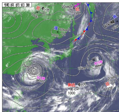
■衛星赤外画像と地上天気図（令和8年8月9日03時）
