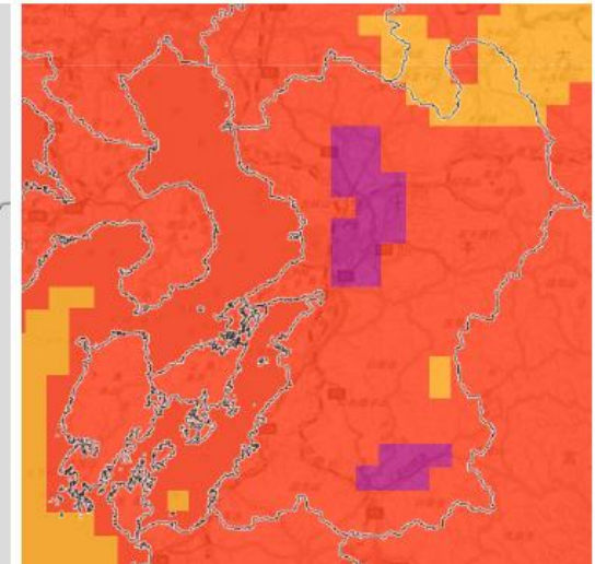
12日 最高気温 (予想)
