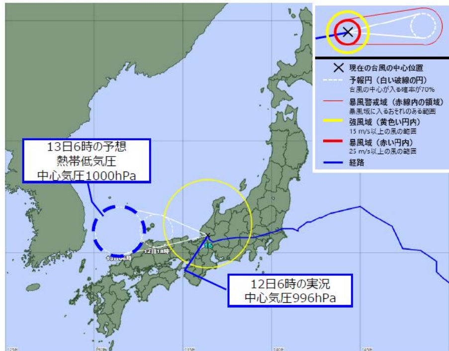
台風第15号 台風経路図 (12日6時時点)
