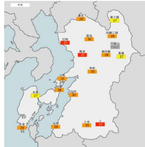
12日 日最高暑さ指数 (予測)
