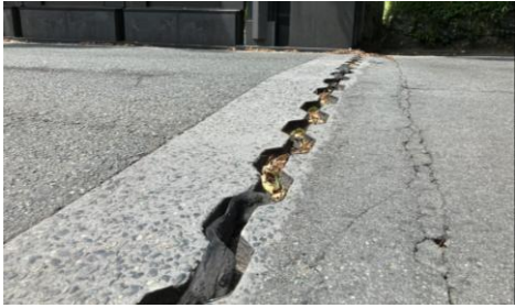
桜橋(伸縮装置の遊間異状)
