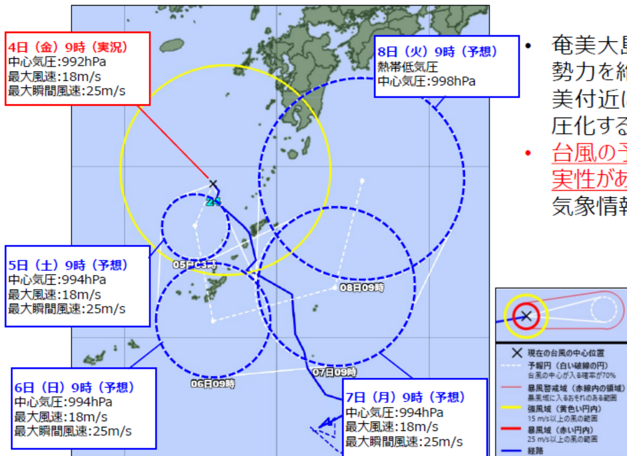
台風経路図（4日9時現在）
