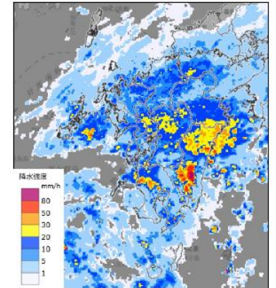
■雨雲の動き（4日10時30分）
