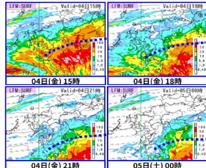
■4日の雨の予想（前3時間降水量、ミリ）
