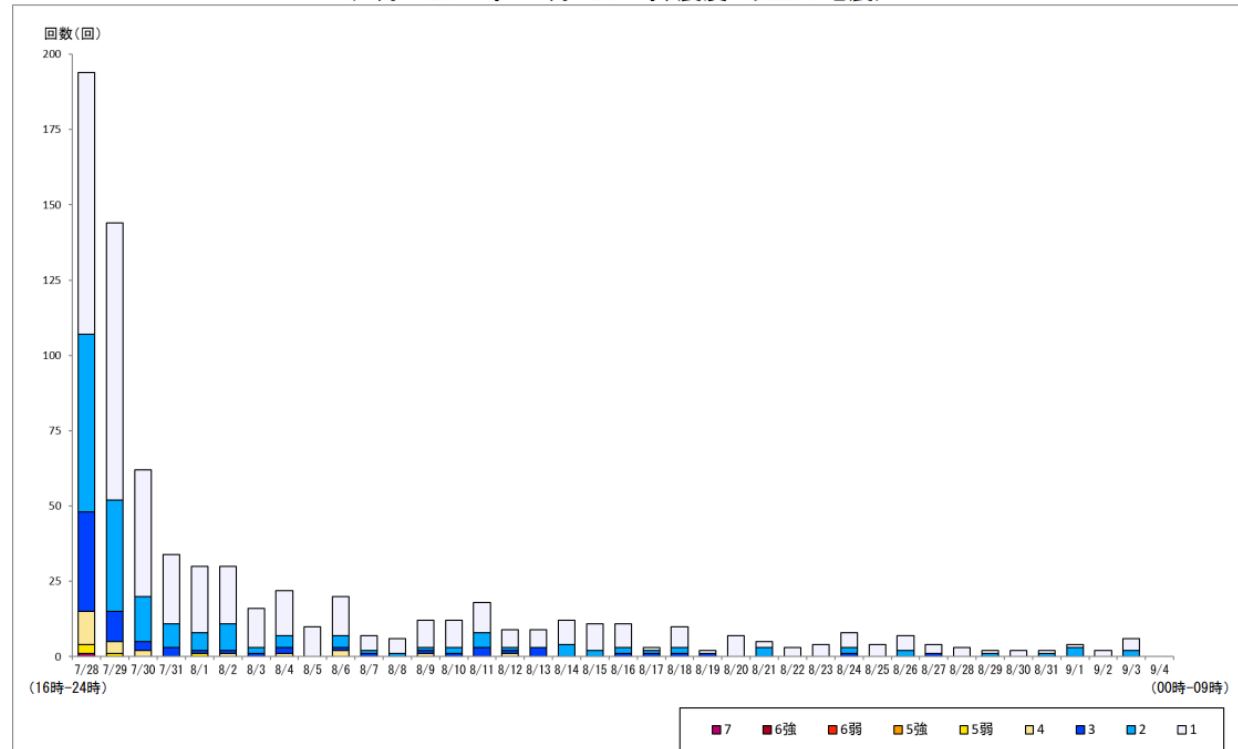
【日別地震回数図】 （7月28日16時～9月4日9時、震度1以上の地震）
