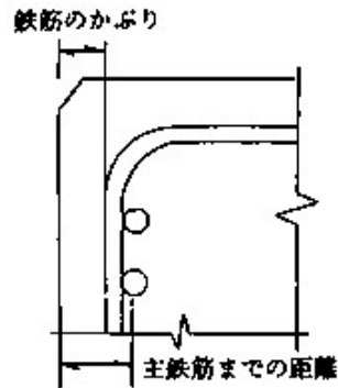
図5-1 鉄筋のかぶり
