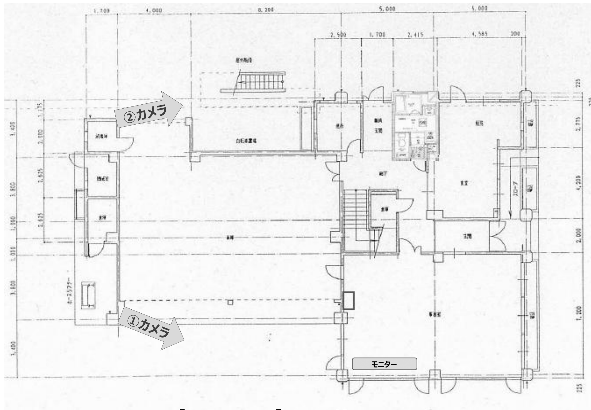
(平面図) 1階
