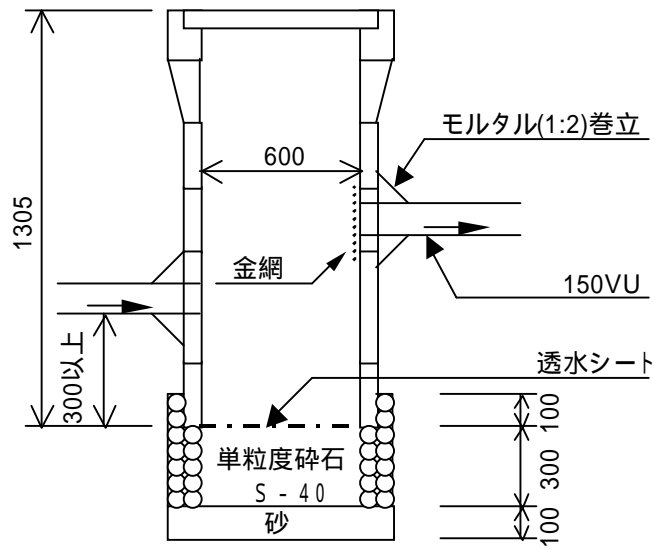
図 7-5 雨水浸透柵標準構造図
