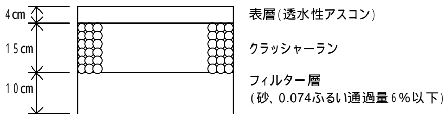
図 7-7 透水性舗装標準構造図
