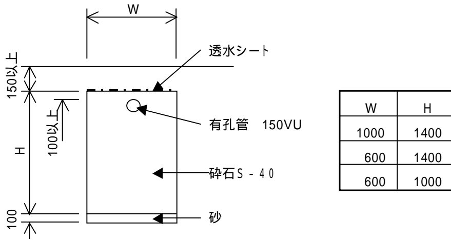
図 7-4 雨水浸透トレンチ標準構造図
