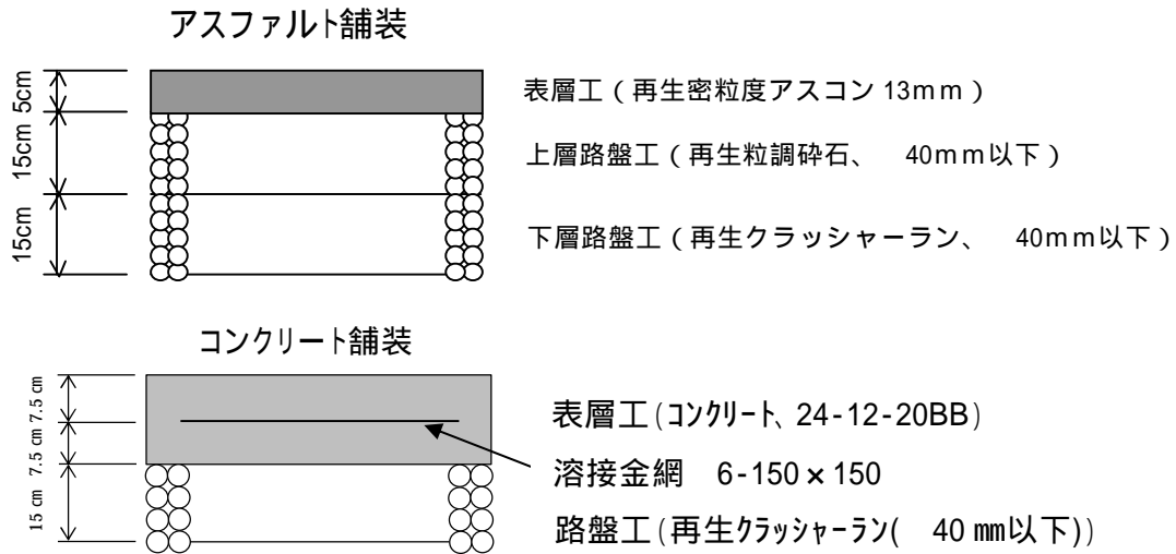
図 4-4 車道舗装標準図
