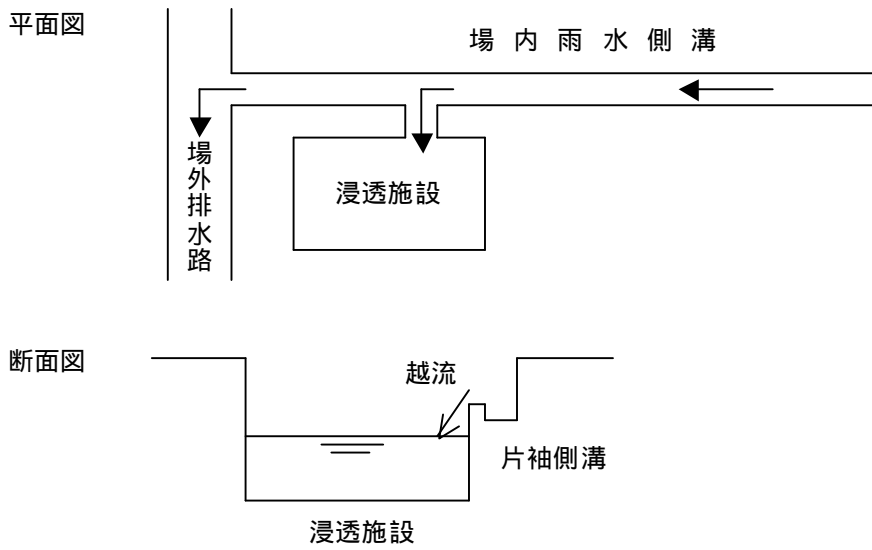
図 7-6 降雨初期流出水の排出例
