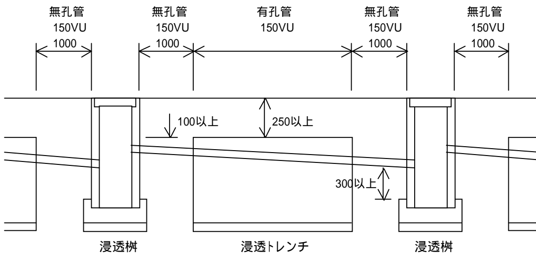
図 7-3 雨水浸透施設の標準図
