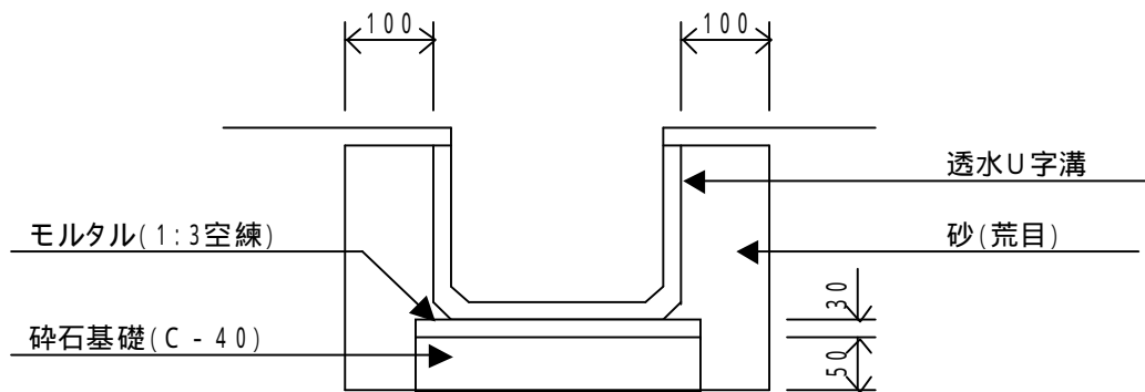
図 7-3 雨水浸透施設の標準図
