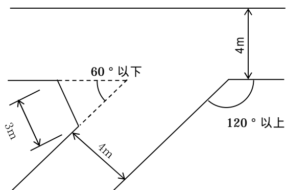
図 4-10 平面交差 例
