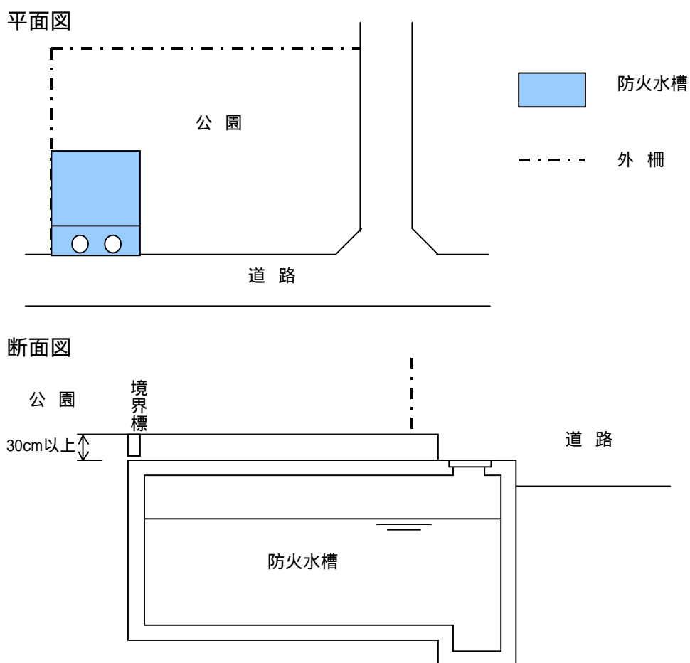
図 5-4 公園と防火水槽を併設する場合の標準図
