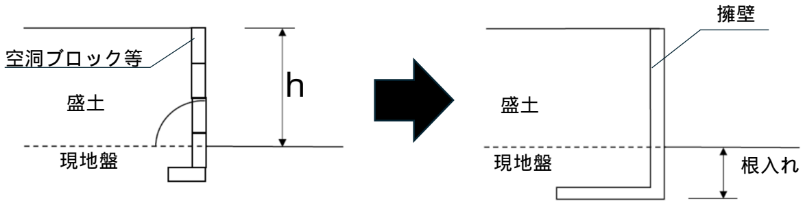
図4.1-1 擁壁の設置が必要な例
