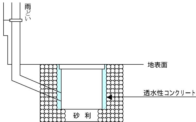
図 7-1 家庭用雨水浸透柵標準図
