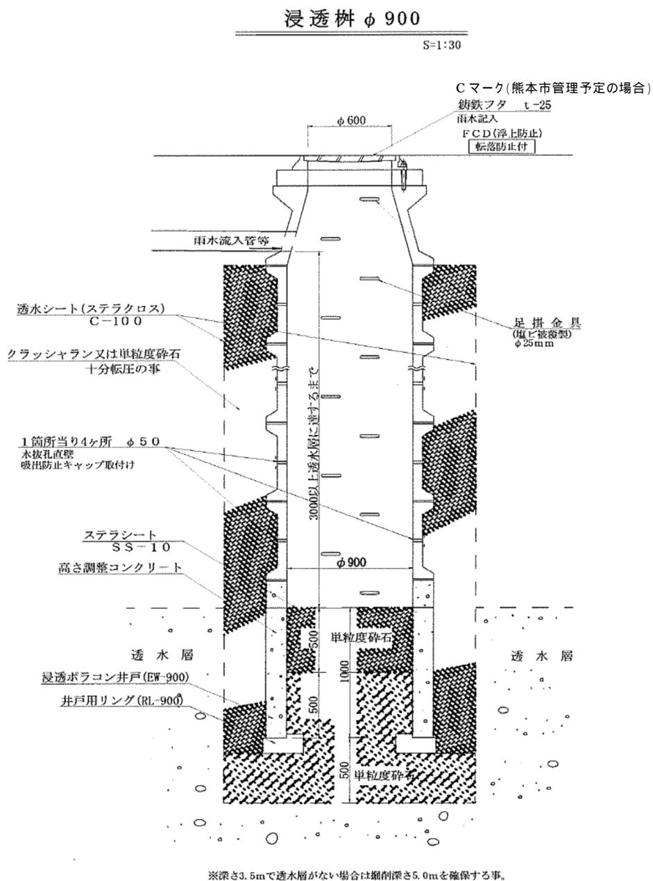
図 7-8 吸込槽標準図(流末がなく 1 宅地面積が 500 m 2 以上の場合)
