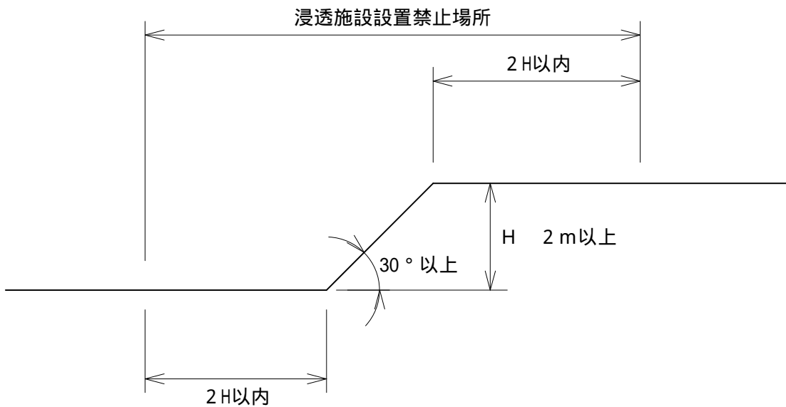
図 7-10 斜面近傍の設置禁止場所の目安
