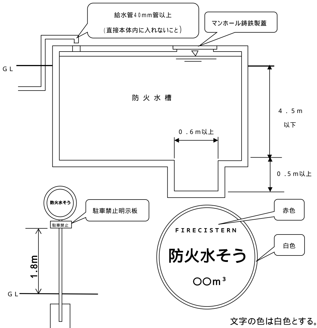
図 10-1 防火水槽標準図
