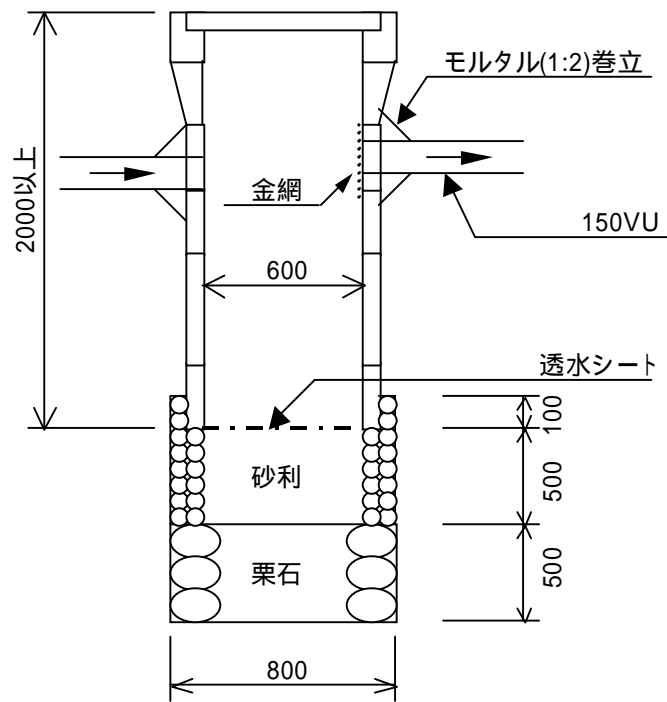
図 7-9 吸込槽標準図(流末がなく 1 宅地面積が 500 m 2 程度の場合)
