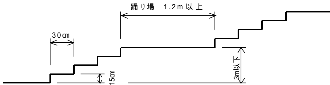
図 4-7 階段道路
