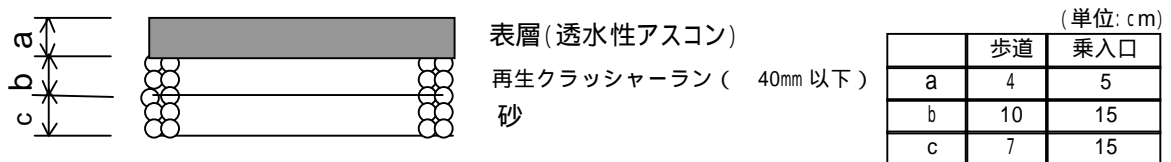
図 4-5 歩道舗装標準図
