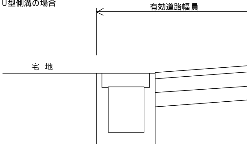
図 4-3 道路幅員
